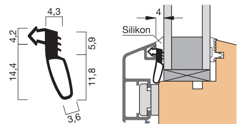
Profilquerschnitt 31197 (M 1:1)
