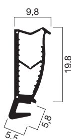
Profilquerschnitt 1042 (M 1:1)
