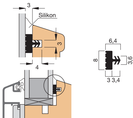
Einbauskizze 2928 (M 1:1)
