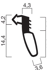
Profilquerschnitt 31197 (M 1:1)
