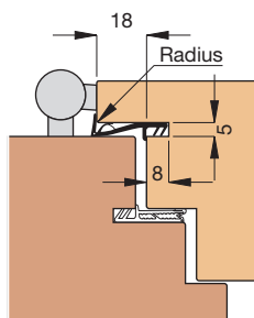
Einbauskizze 1031 (M 1:3)
