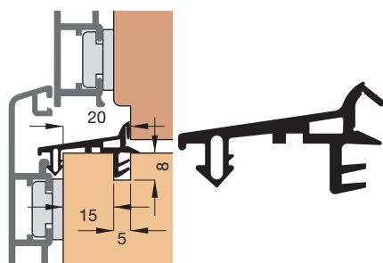
Einbauskitze 31190 (M 1:2)
