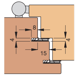
Einbauskizze 1028 (M 1:3)
