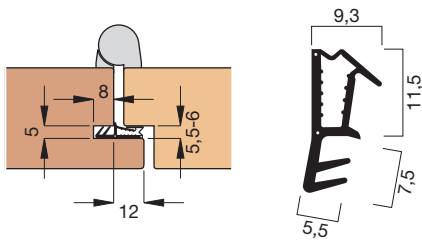
Einbauskizze 1044 (M 1:3)
