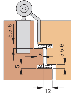
Einbauskizze 1044 (M 1:3)
