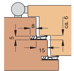
Einbauskizze 1038 (M 1:3)
