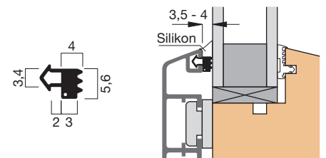
Profilquerschnitt 31264 (M 1:1)
