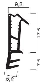
Profilquerschnitt 1046 (M 1:1)
