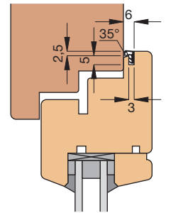
Einbauskizze 2611 (M 1:3)
