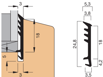
Einbauskizze 2914 (M 1:1)
