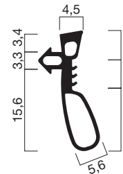
Profilquerschnitt 31171 (M 1:1)
