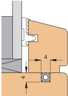
Einbauskizze Einbau im Fensterflügel 2931 (M 1:1)
