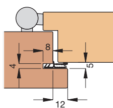
Einbauskizze 1036 (M 1:3)
