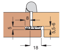
Einbauskizze 1046 (M 1:3)
