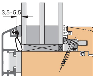
Einbauskizze Fixverglasung 31208 (M 1:2)
