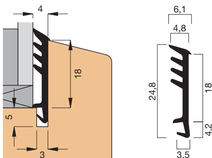
Einbauskizze 2915 (M 1:1)
