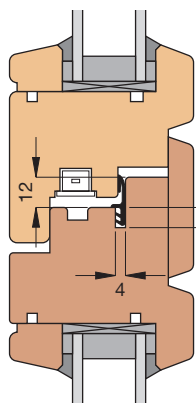
Einbauskizze 2044 (M 1:3)
