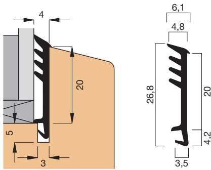
Einbauskizze 2913 (M 1:1)
