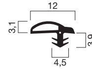
Profilquerschnitt 2057 (M 1:1)
