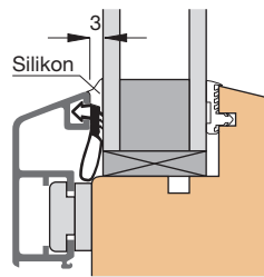
Einbauskizze 31391 (M 1:2)
