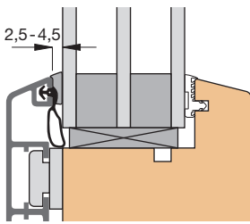
Einbauskizze 31207 (M 1:2)
