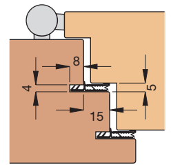
Einbauskizze 1037 (M 1:3)
