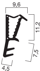
Profilquerschnitt 1036 (M 1:1)
