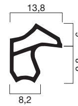
Profilquerschnitt 1602 (M 1:1)
