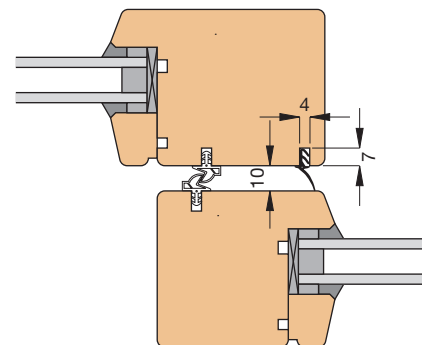
Einbauskizze 9018 (1:3)
