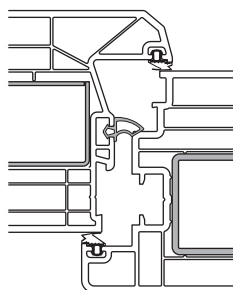
Einbauskizze 3550 (M 1:3)
