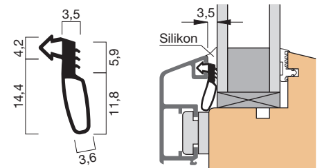
Profilquerschnitt 31125 (M 1:1)
