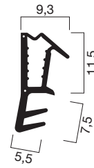
Profilquerschnitt 1044 (M 1:1)
