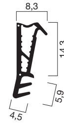
Profilquerschnitt 1028 (M 1:1)
