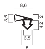
Profilquerschnitt 31279 (M 1:1)
