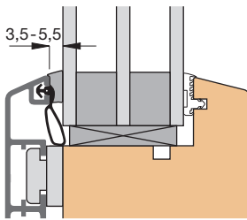
Einbauskizze 31208 (M 1:2)
