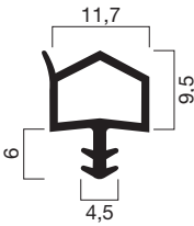
Profilquerschnitt 1007 (M 1:1)
