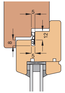
Einbauskizze 2001 (M 1:3)
