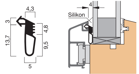
Profilquerschnitt 3183 (M 1:1)
