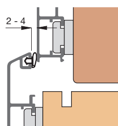
Einbauskizze 3153 (M 1:2)
