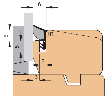
Profilquerschnitt 2807 (M 1:1)
