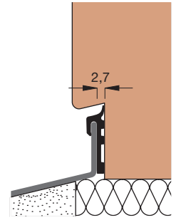
Einbauskizze 2060 (M 1:2)
