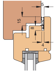
Einbauskizze 2603 (M 1:3)
