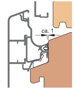
Einbauskizze 31317 (M 1:2)
