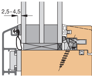
Einbauskizze Fixverglasung 31207 (M 1:2)
