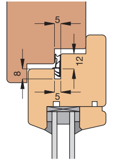
Einbauskizze 2003 (M 1:3)
