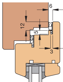
Einbauskitze 2054 im Überschlag (M 1:3)
