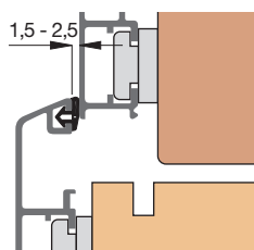
Einbauskizze 2045 (M 1:2)
