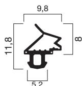
Profilquerschnitt 3550 (M 1:1)
