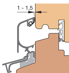
Einbauskizze 31151 (M 1:2)
