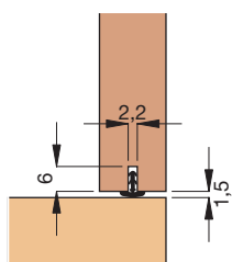
Einbauskizze 4001 (M 1:2)
