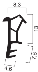
Profilquerschnitt 2030 (M 1:1)
