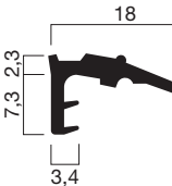
Profilquerschnitt 9022 (M 1:1)
